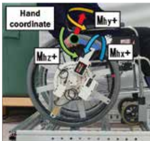
図1 操作力計測用の車いす
