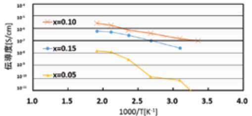
図 Sn 1-x Al x P 2 O 7 (x=0.05, 0.10, 0.15) の伝導度のアレニウスプロット
