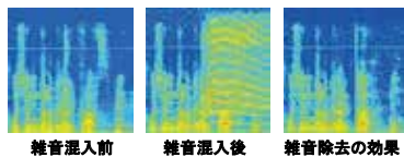
図2 雑音除去手法による効果
