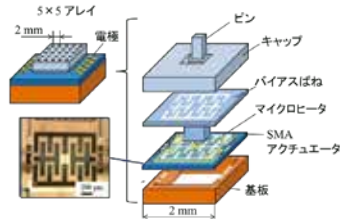
図 1 形状記憶合金を用いた触覚ディスプレイ
