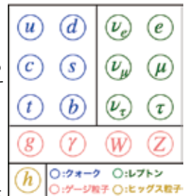
図 1 素粒子の種類
