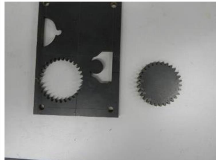
射出ワイヤカット放電加工機
