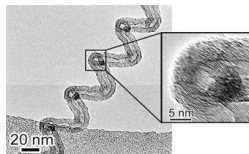
多層カーボンナノコイル
