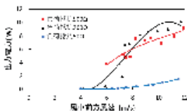
図2 風車の出力特性
