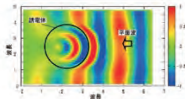
図3 FDTD 法による計算例
