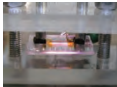
図2 マイクロチップ内の He プラズマ
