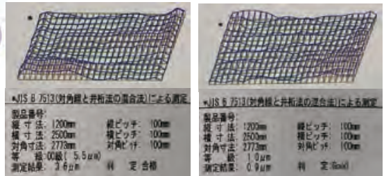
図 2. ハンドラップによる平面精度の向上
