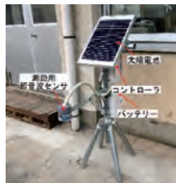
図3 独立電源式
