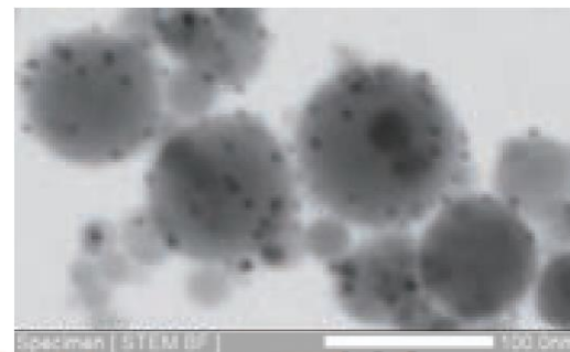
TiO 2 粒子上の銀ナノ粒子
